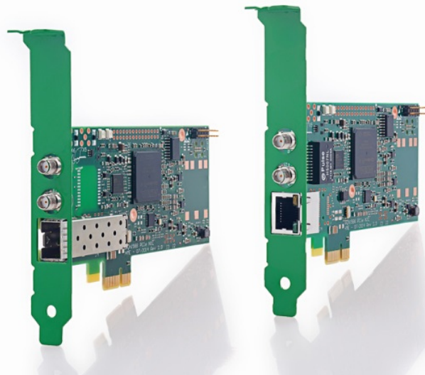
syn1588® PCIe NIC Revision 2
